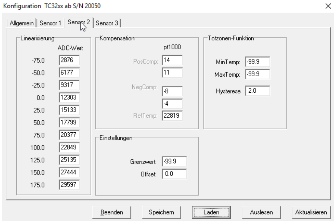
Konfigurations-Dialog - Sensor 2 (je nach Firmware-Version kann ein Teil der Werte entfallen)
