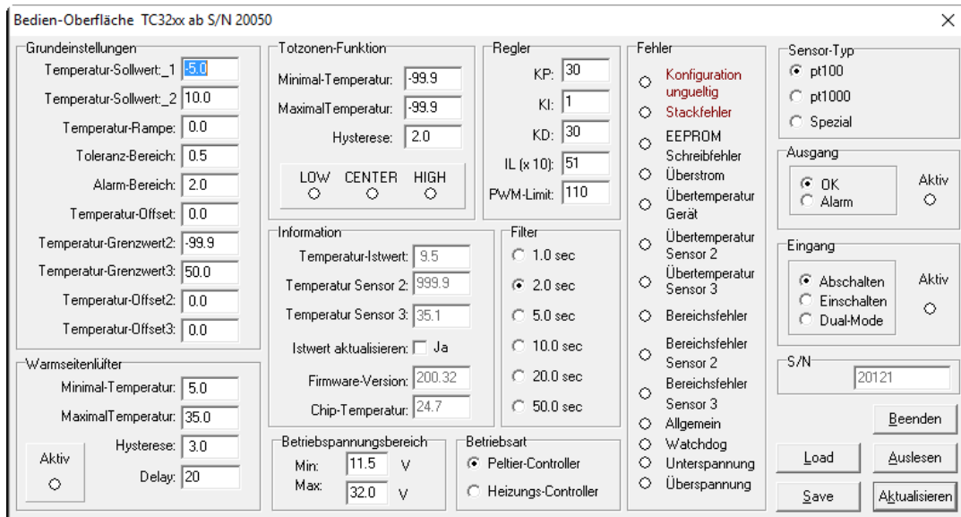
Bedien-Oberfläche TC3224
