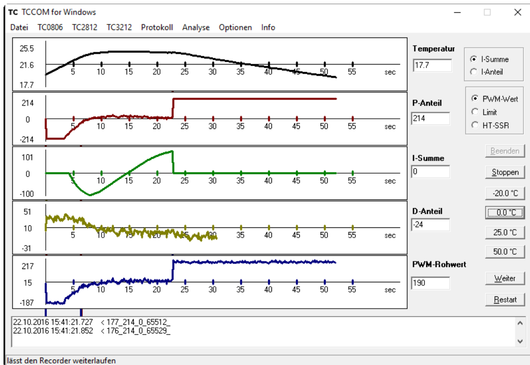
Recorder-Anzeige
