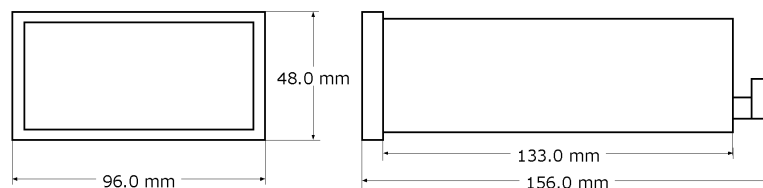
Schalttafel-Ausschnitt: 92.5 mm x 43 mm
